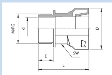
Plastový konektor ; neohebný pripojovací závit
